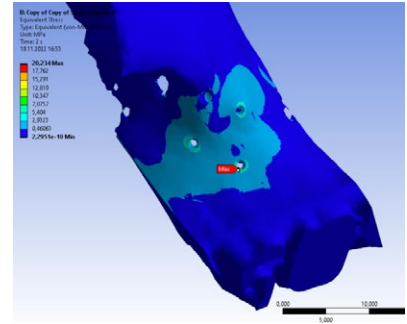
Рис. 12. Максимально эквивалентное напряжение у ортодонтического винта составило 20,2 МПа Fig. 12. The maximum equivalent stress at the orthodontic screw was 20.2 MPa
